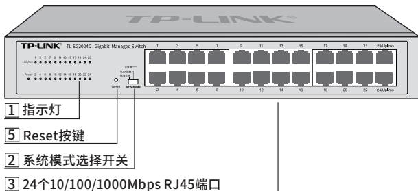
图1-5 TL-SG2024D前面板示意图
